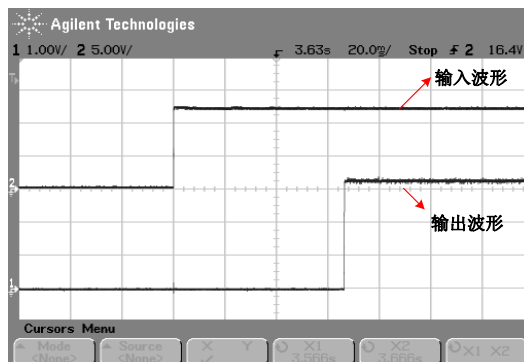
图 2.5 启动波形
