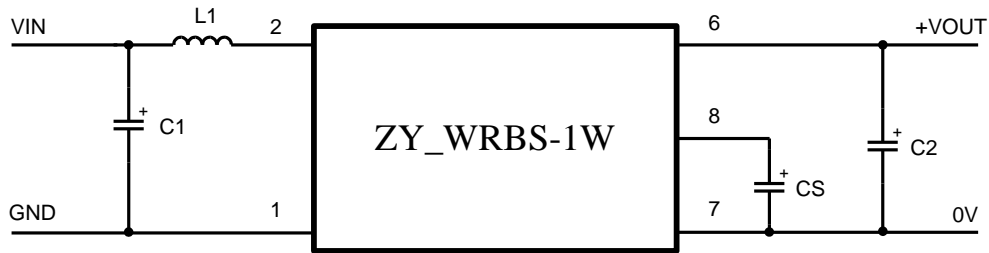
图 4.1 ZY_WRBS-1W 接口电路
