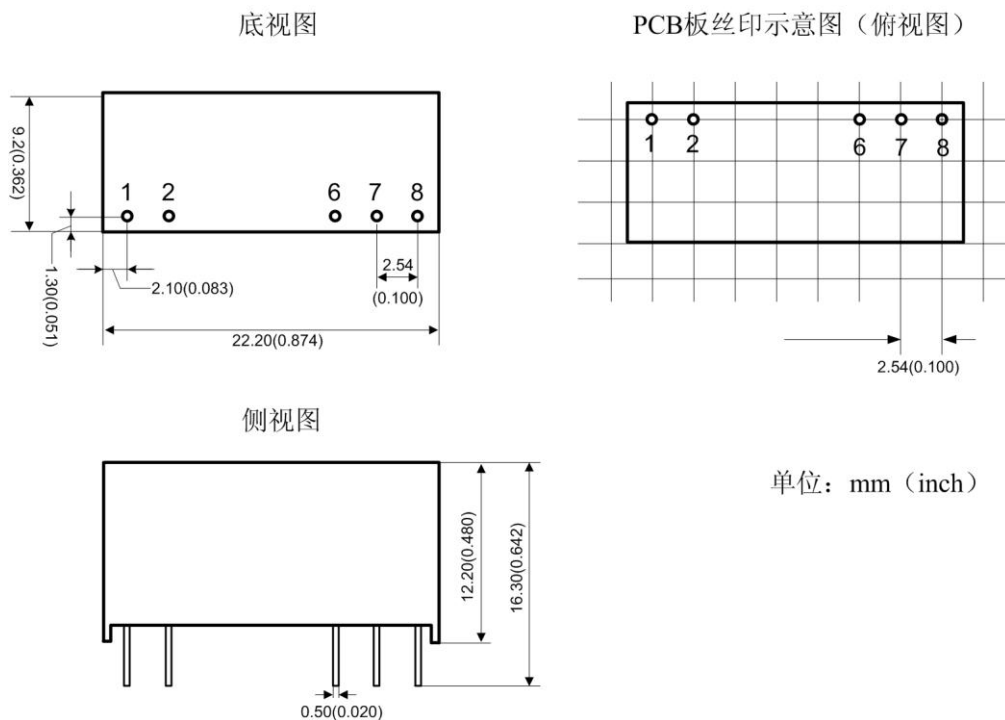
图 6.1 ZY_WRBS-1W 机械尺寸图
